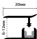
ПОРОГ ДЛЯ ЛАМИНАТЫ ПРИСТЕННЫЙ С ФИКСАТОРОМ
