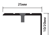
УГОЛ-ПОРОГ 25MMX10MM/20MM
