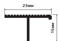
ПРОФИЛЬ РИФЛЕННЫЙ ДЛЯ СТУПЕНИ
