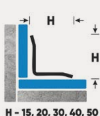
ВНУТРЕННИЙ УГОЛ
